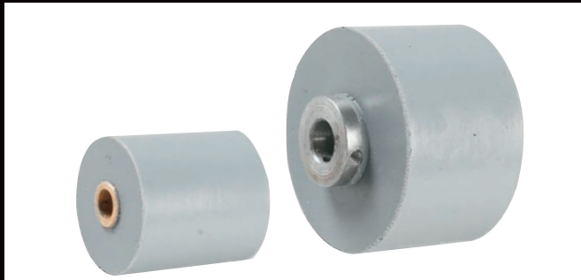
Nouveaux galets d'alimentation et rouleau entraineur de 38mm en uréthane, assurant en meilleur entrainement et défilement de la bande gommée et la régularité de la vitesse de la bande
